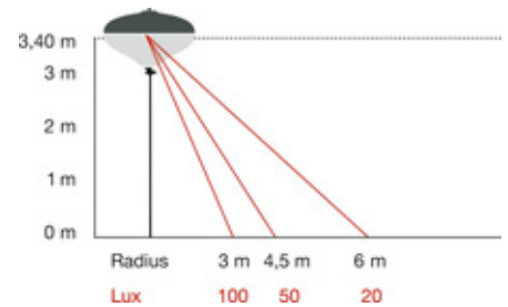
Illuminazione con lampada alogena e treppiede con 3,4 metri di altezza
