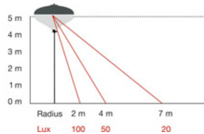
Illuminazione con lampada alogena e treppiede con 5 metri di altezza
