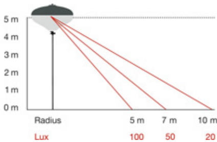
Illuminazione con lampada HQI e treppiede con 5 metri di altezza
